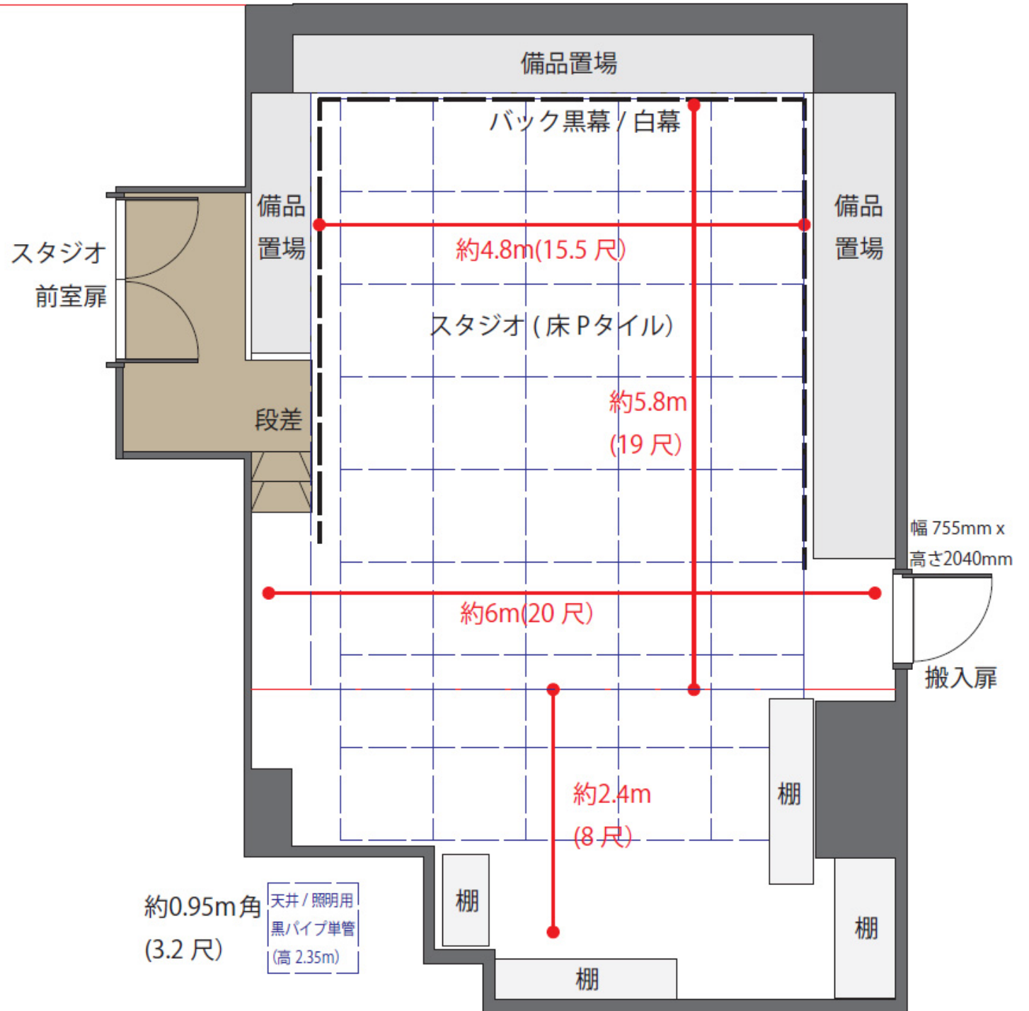
(平面図)
